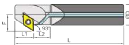
Coolant carbide shank (right shown) 中心出水鎢鋼柄 右向示意圖
