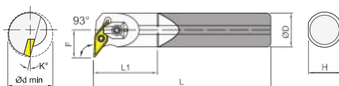
Carbide shank+clamp (right shown) 錫鋼柄+壓板 右向示意圖
