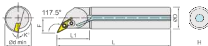
Coolant steel shank+clamp (right shown) 中心出水鋼柄+壓板 右向示意圖
