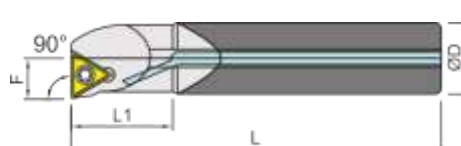
Coolant carbide shank (right shown) 中心出水鎢鋼柄 右向示意圖
