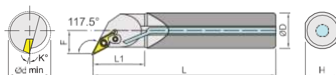
Coolant carbide shank+clamp (right shown) 中心出水鎢鋼柄+壓板 右向示意圖
