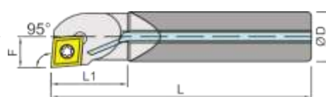
Coolant carbide shank (right shown) 中心出水鎢鋼柄 右向示意圖
