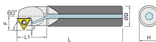
Coolant carbide shank (right shown) 中心出水鎢鋼柄 右向示意圖
