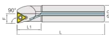
Coolant steel shank (right shown) 中心出水鋼柄 右向示意圖
