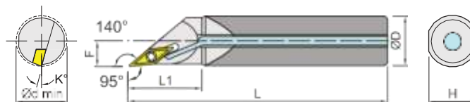
Coolant carbide shank (right shown) 中心出水鋁鋼柄 右向示意圖
