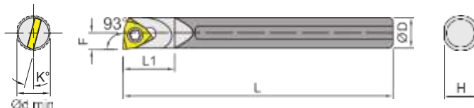
Carbide shank (right shown) 錫鋼柄 右向示意圖
