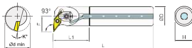
Coolant steel shank+clamp (right shown) 中心出水鋼柄+壓板 右向示意圖
