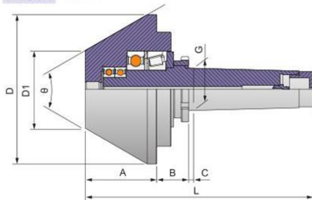
尺寸表 單位: mm
